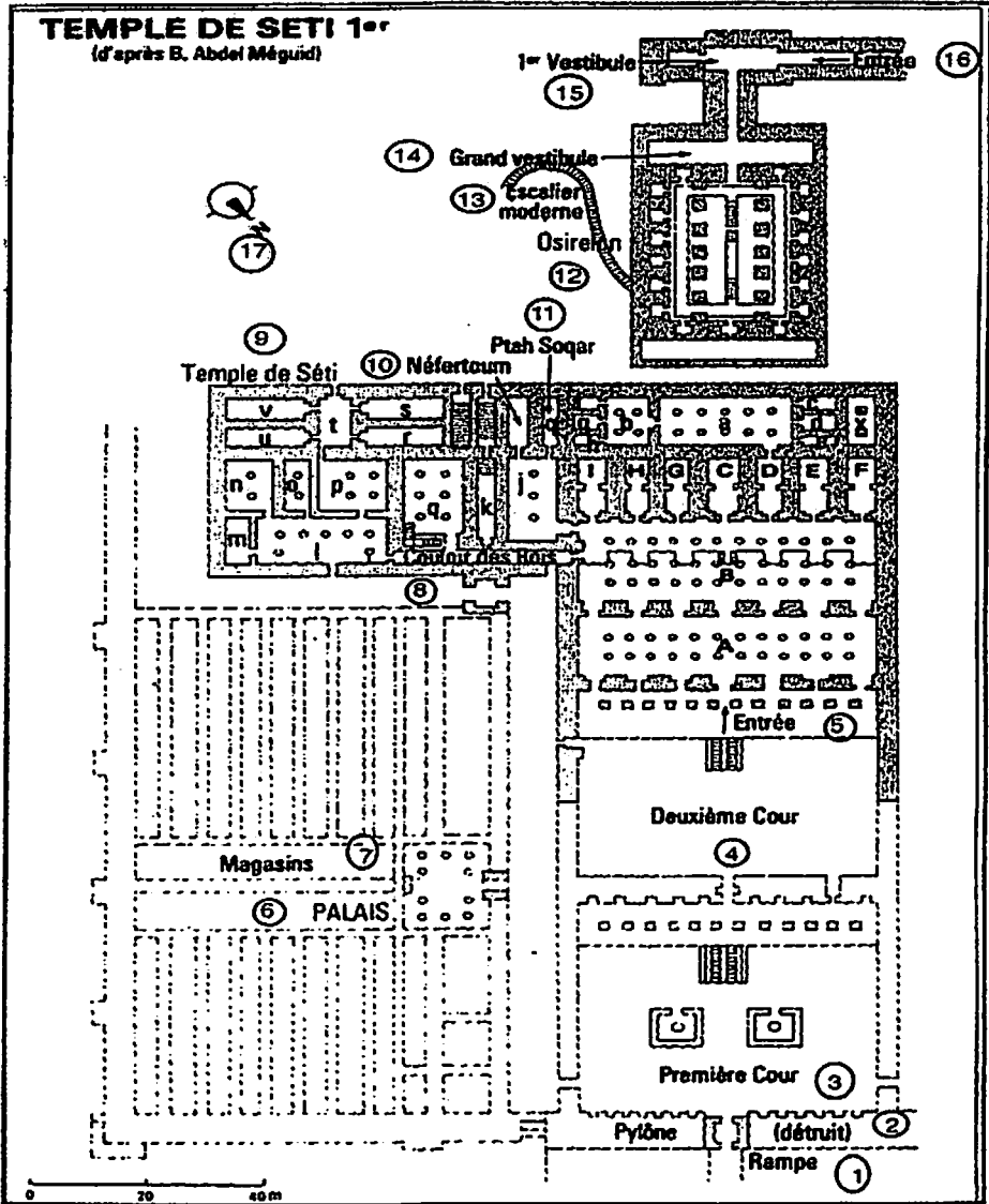
مسقط أفقى لمعبد سيتى الأول ، فى أبيدوس
